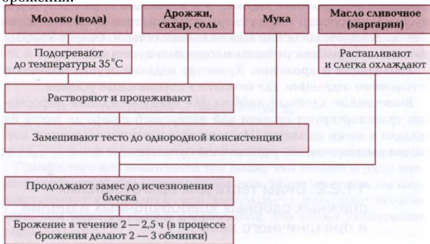
Рис. 11.1. Технологическая схема приготовления дрожжевого безопарного теста
