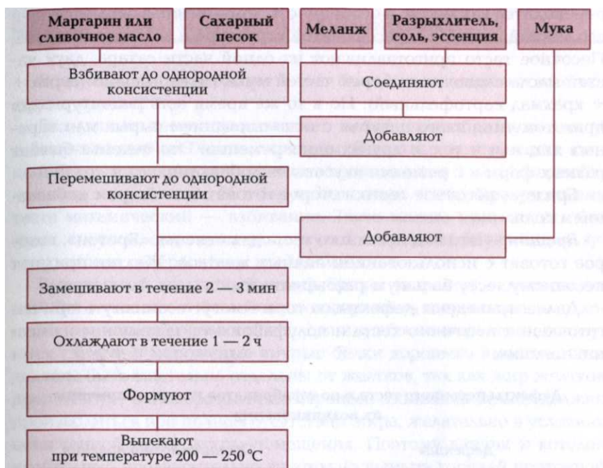
Рис. 14.4. Технологическая схема приготовления песочного полуфабриката
